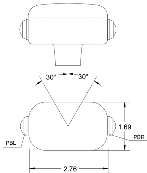
MG13 dimensions
