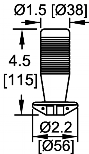
RH dimensions
