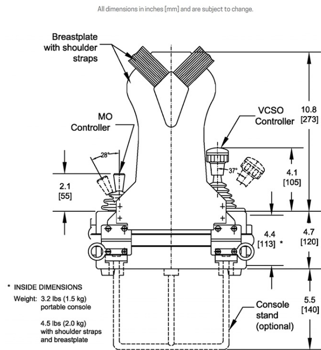
FGC-01-A dimensions
